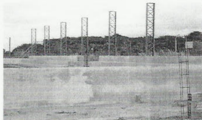
Foto 6 – Piso do degrau da arquibancada que foi alterado ao projeto original – quadra Monte Cristo
