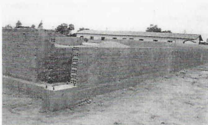
Foto 13- Quadra do Bairro Sen. Hélio Campos
